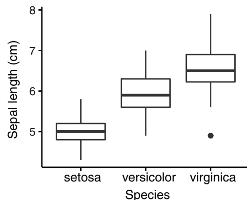
図2 アヤメ3種における萼片の長さ
