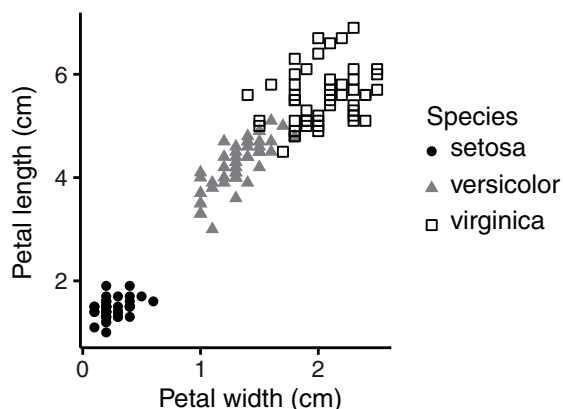
図1 アヤメ3種の花弁の幅と長さの散布図
